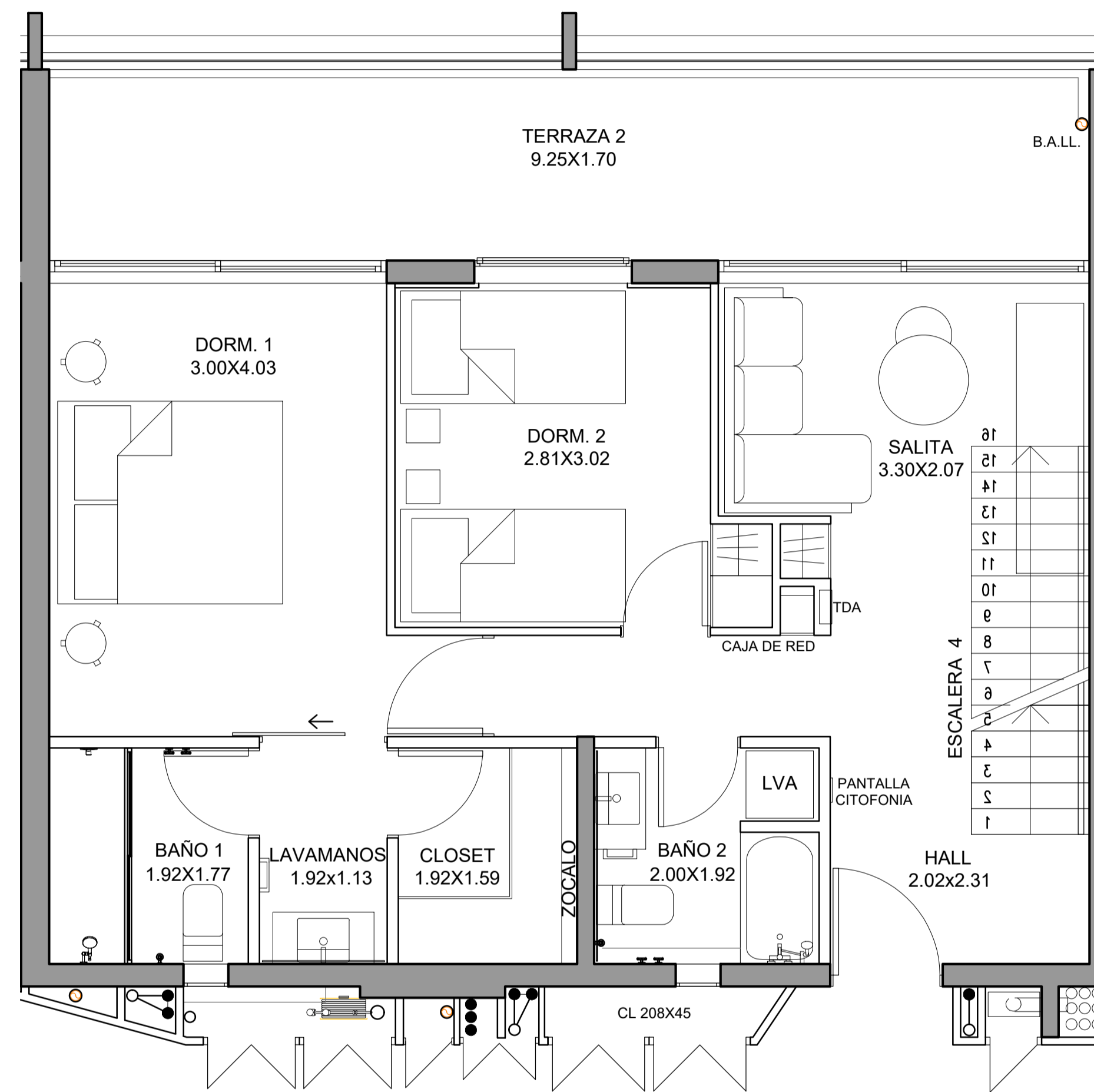
DEPARTAMENTO TIPO B1 NIVEL ACCESO
