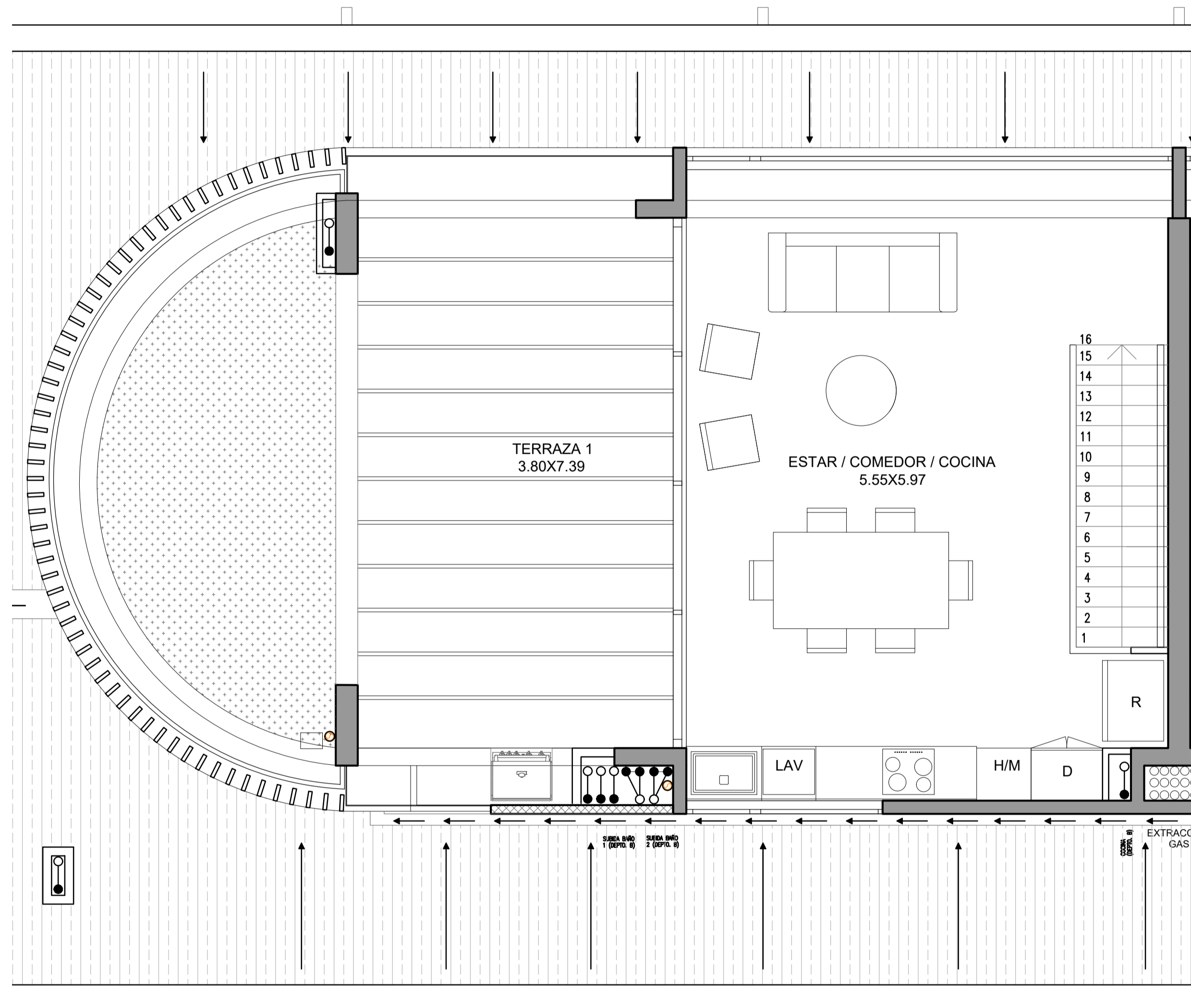
DEPARTAMENTO TIPO B1 NIVEL 2
